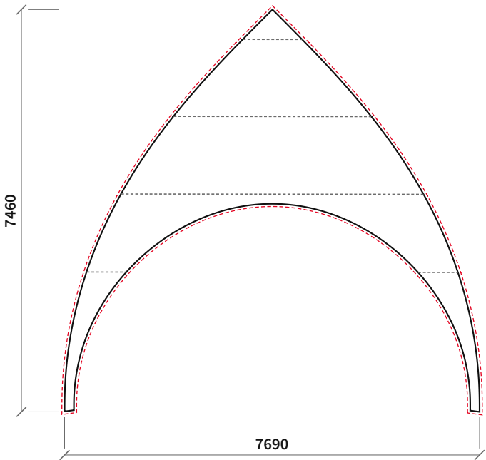
EINZELSEGMENT, MASSSTAB 1:100
