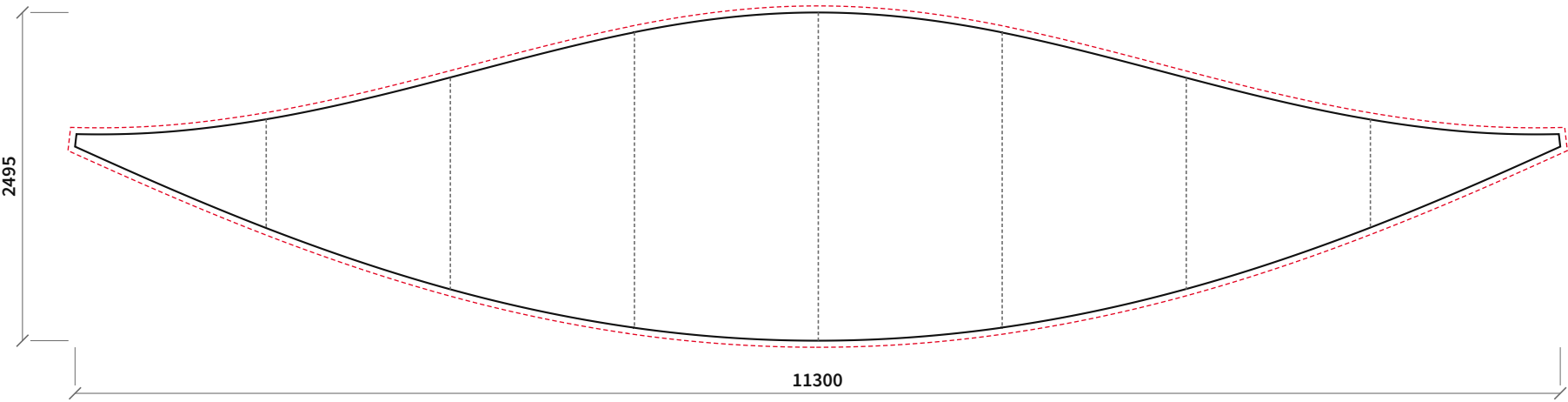
EINGANGSBOGEN, MASSSTAB 1:50
